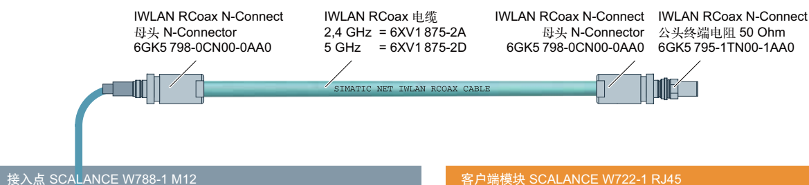
接入点 SCALANCE W788-1 M12
