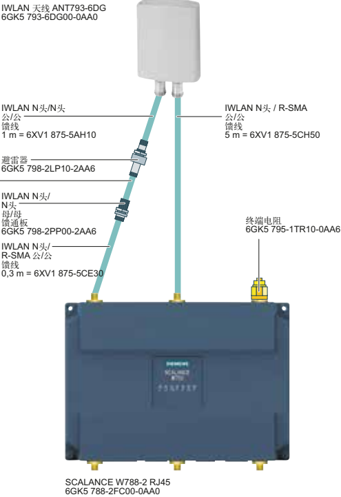
双斜面天线 ANT793-6DG 通过 R-SMA 端口连接至 SCALANCE W788-2 RJ45
