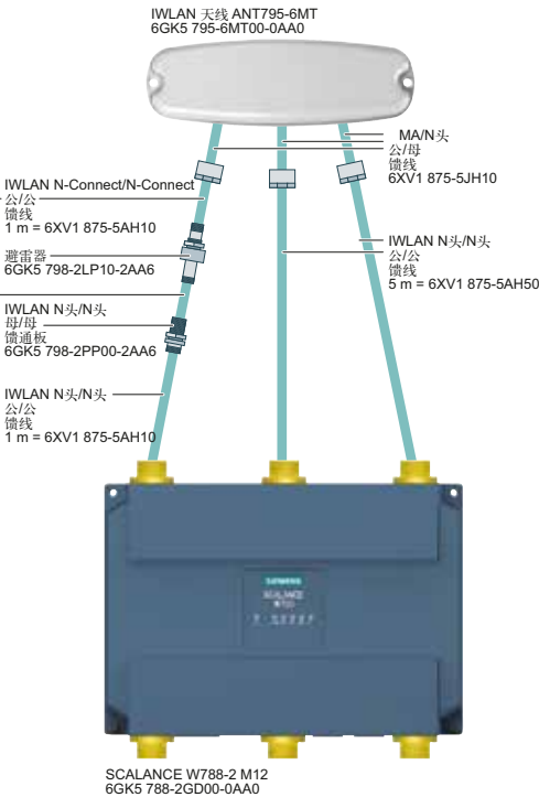
MIMO 天线 ANT795-6MT 通过 N-Connect 端口连接至 SCALANCE W788-2 M12
