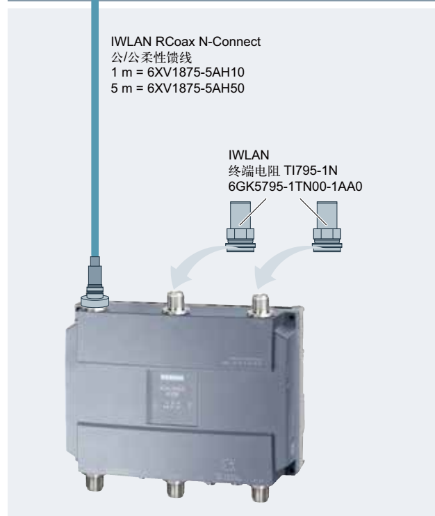
接入点 SCALANCE W788-1 M12
