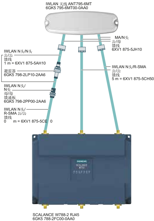
MIMO 天线 ANT795-6MT 通过 R-SMA 端口连接至 SCALANCE W788-2 RJ45
