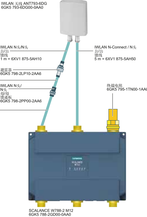
双斜面天线 ANT793-6DG 通过 N-Connect 端口连接至 SCALANCE W788-2 M12
