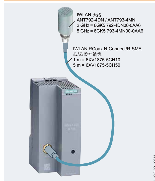
客户端模块 SCALANCE W722-1 RJ45
